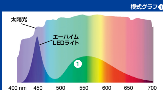
太陽光とエーハイム LEDライト①の波長スペクトル
